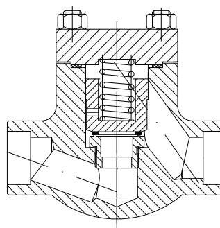
Piston Type
