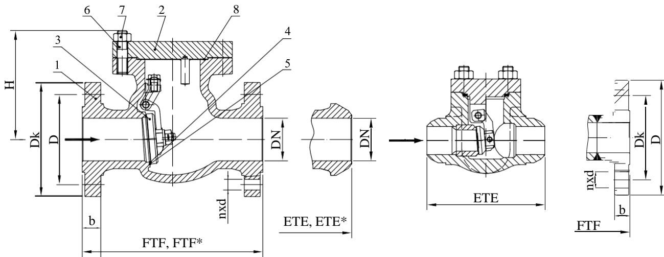
Rysunek B.2.1 Części i wymiary
