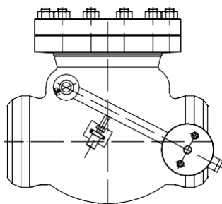
Zawór zwrotny z przeciwwagą
