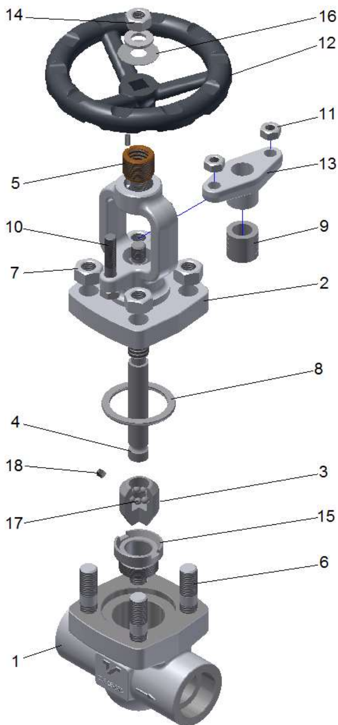
Rysunek 1. Części składowe kątego zaworu zaporowego
