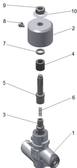
Rysunek 1. Części składowe zaworu i lista części zamiennych.
