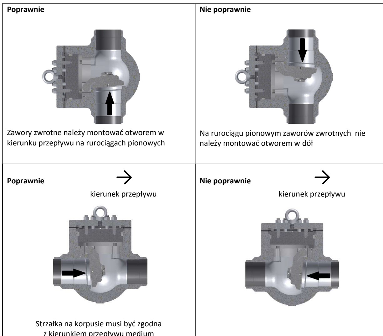
Rysunek 3. Dozwolona pozycja montażu
