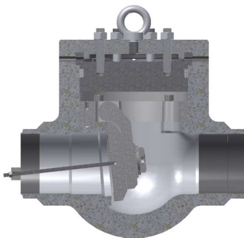
Rysunek 2. Zawór zwrotny klapowy z zabezpieczeniem dysku
