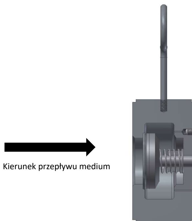
Rysunek 2. Dozwolona pozycja montażu
