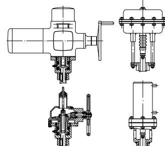
Upravljanje električno, reduktorom, pneumatsko ili hidraulično
