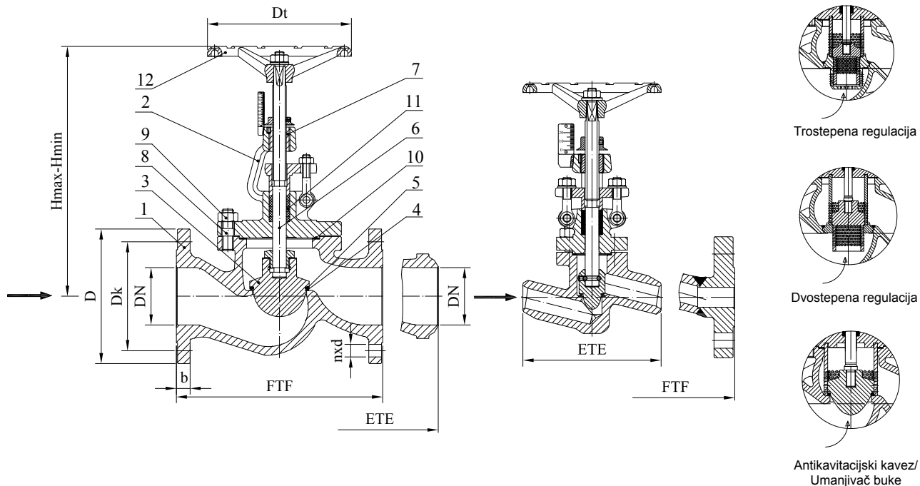
Crtež A.2.1 Pozicije i mere
