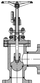
Ugaoni tip [VENRA]
