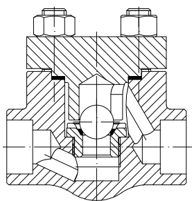
Kovani odbojni ventil sa kuglom
