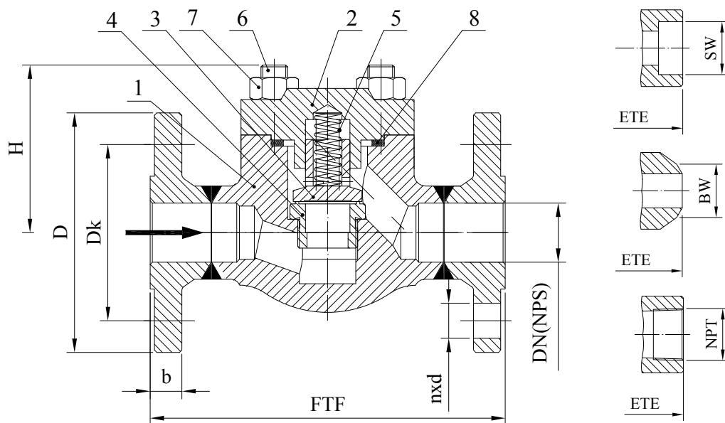
Crtež B.5.1 Pozicije i mere
