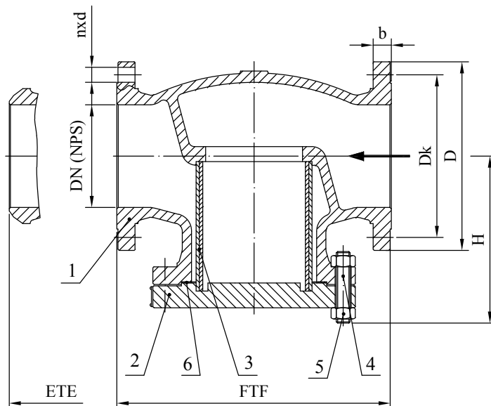
Crtež C.2.1 Pozicije i mere
