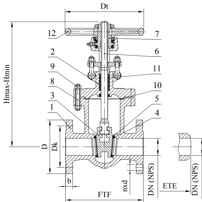
Crtež D.2.1 Pozicije i mere
