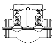
Sa by-pass ventilima i rasteretnim vodom
